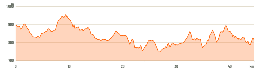
Altitude ao longo do ramal Guaxupé – Caconde, em quilômetros acumulados. Cada risco embaixo é o fim de uma etapa. Altitude lida por nós no modelo de terreno ANADEM.
